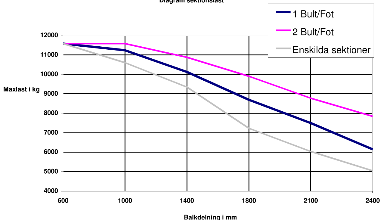
Diagram sektionlast
